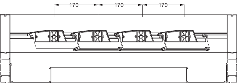
Lame big - Rotazione lamelle a 0°
