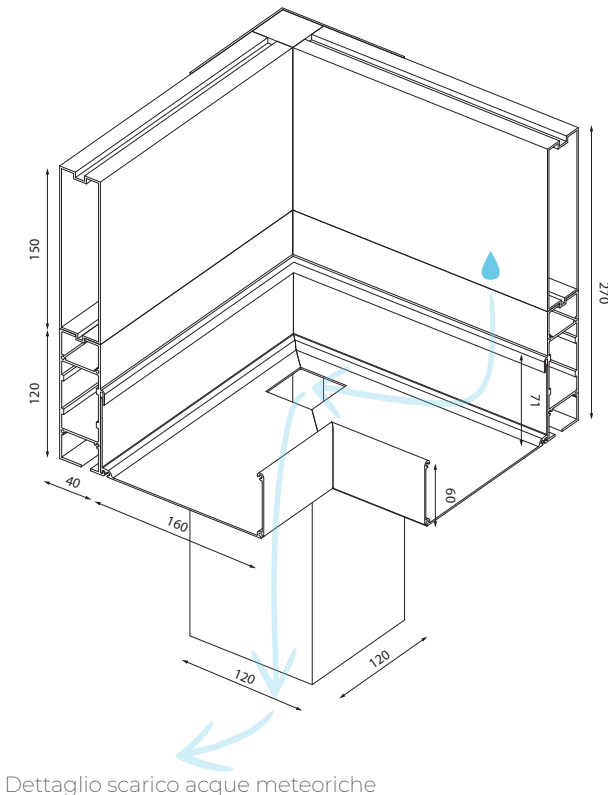
Dettaglio scarico acque meteoriche
