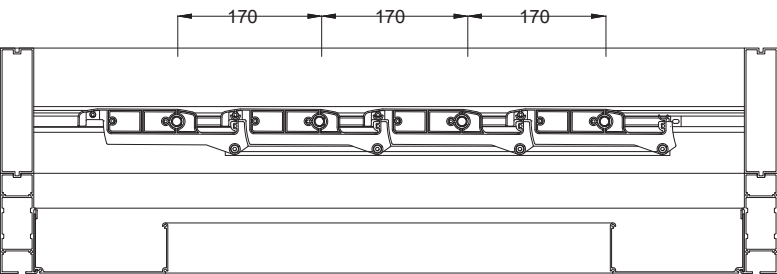
Lame slim - Rotazione lamelle a 0°
