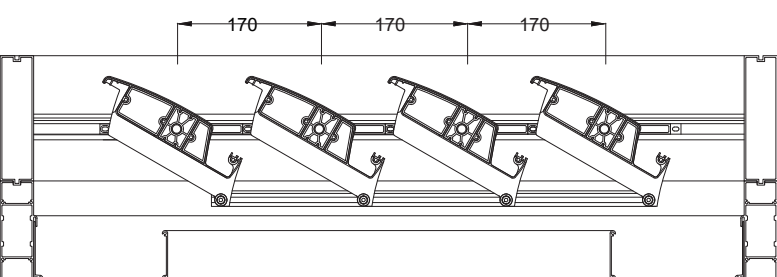
Lame big - Rotazione lamelle a 45°
