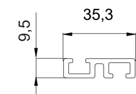
Asta di movimentazione
