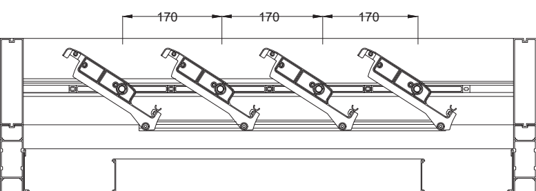
Lame slim - Rotazione lamelle a 45°
