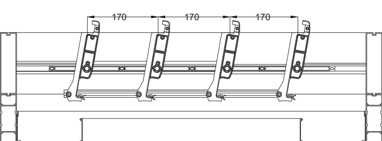
Lame slim - Rotazione lamelle a 100°
