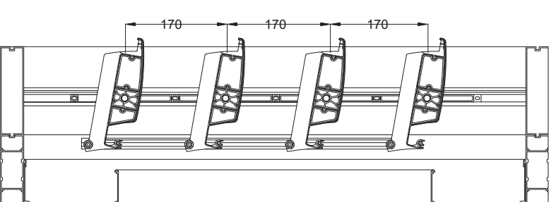
Lame big - Rotazione lamelle a 100°
